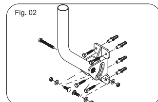
2. Instalação do suporte na parede, fig. 02. 2. Instalación de septn.en la pared fig. 02.
