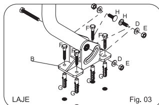
3. Para a antena SHD 8000K, faça a marcação na laje ou parede utilizando o suporte como gabarito e insira as buchas nos furos, fig. 03/04. Fixe o suporte utilizando os parafusos que acompanham o produto.
