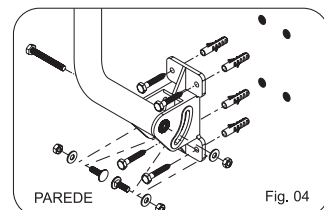
3. Para a antena SHD 8000K, faça a marcação na laje ou parede utilizando o suporte como gabarito e insira as buchas nos furos, fig. 03/04. Fixe o suporte utilizando os parafusos que acompanham o produto.
