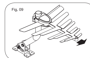
8. Direcione a antena para as torres de transmissão para buscar a melhor recepção de sinal em todos os canais fig 09.
